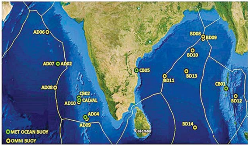
సముద్రంలో సునామీ రాకను తెలిపే 'బూయ్స్' (పసుపు రంగులోనివి)
